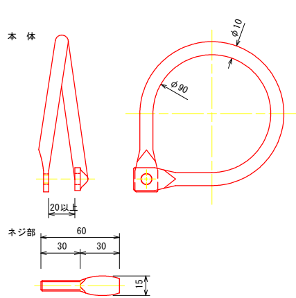
A Zワイヤージョイント (内径90mm)
